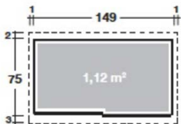
Grundriss Gartenschrank 157
